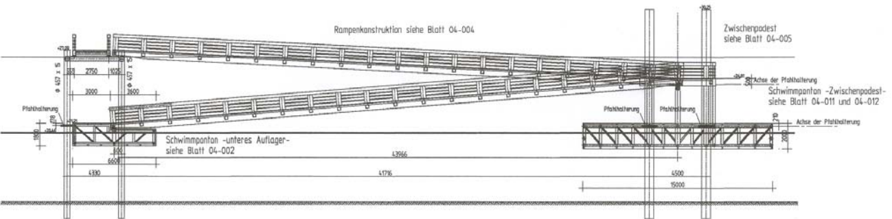
Ansicht Rampenkonstruktion
