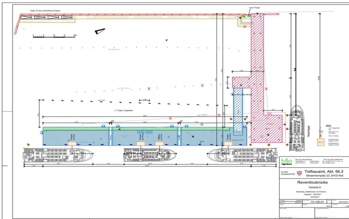
Lageplan Zugang, Rampe und Schwimmponton
