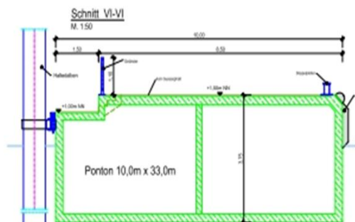
Systemschnitte Zugang auf Gründungspfählen und Schwimmponton an Dalben gehalten
