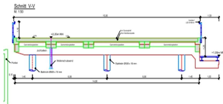
Systemschnitte Zugang auf Gründungspfählen und Schwimmponton an Dalben gehalten
